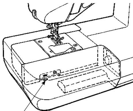
Drop feed knob Transporteurschieber Transporteurknop ручка для регулирования зубчатого двигателя ткани
